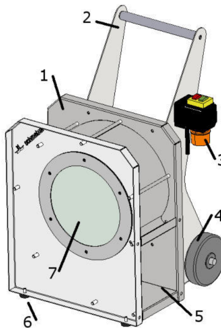
Figura 1: Ventilador tal y como se entrega
