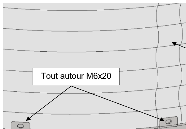
Représentation 12 : Détail de l'étape de montage 5 : Tube extérieur en tôle perforée.
