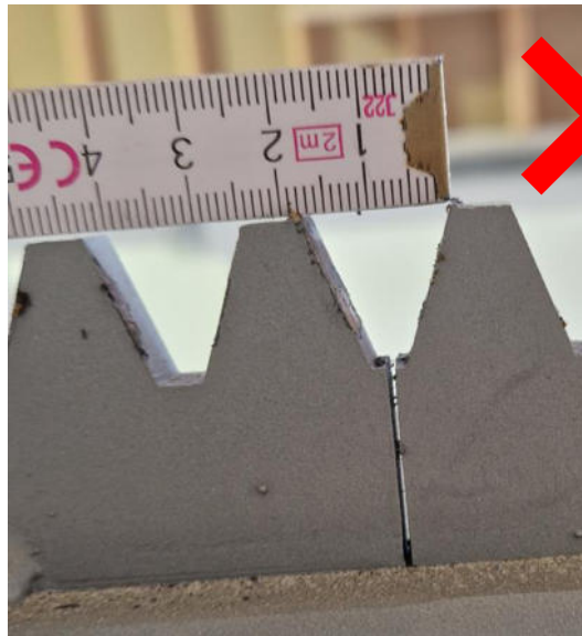
Figura 5: ejemplo incorrecto, la distancia es demasiado corta.
