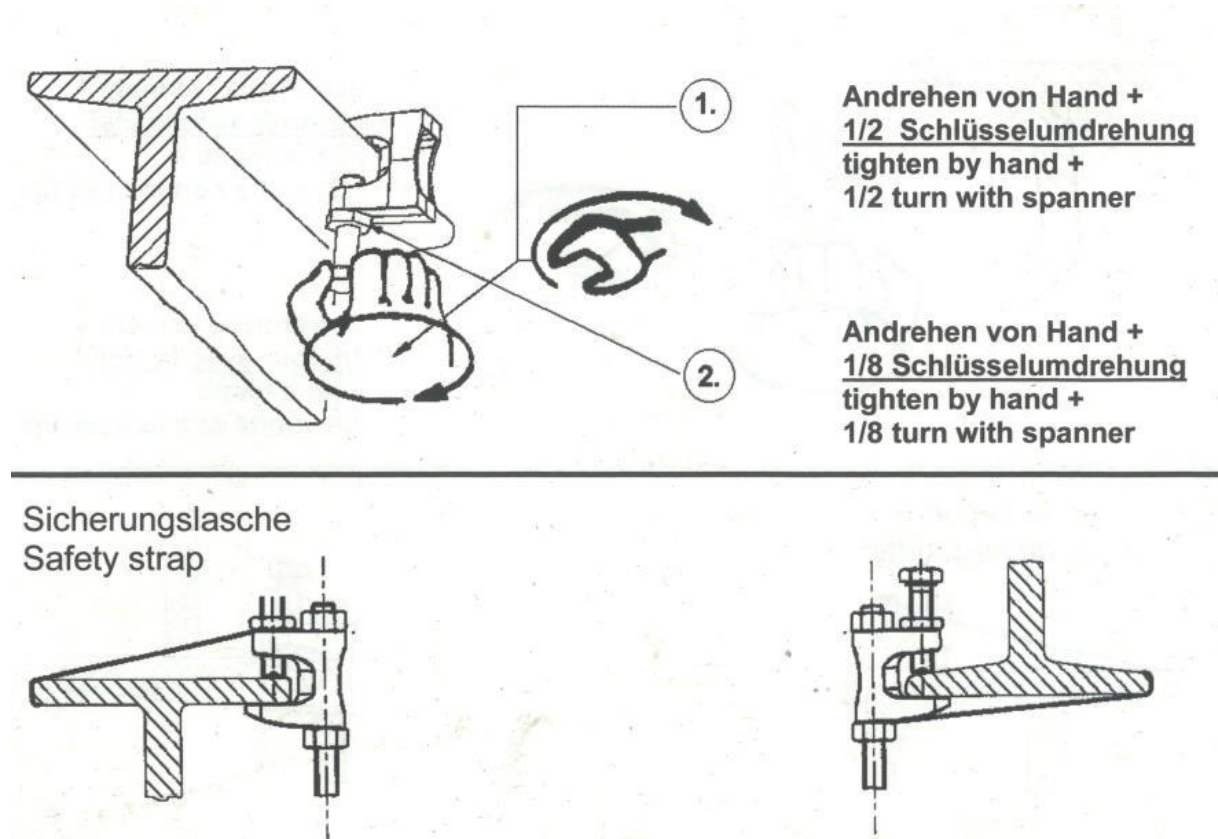
Abbildung 21: Anzug der Trägerklemmen der Endschalterhalter.
