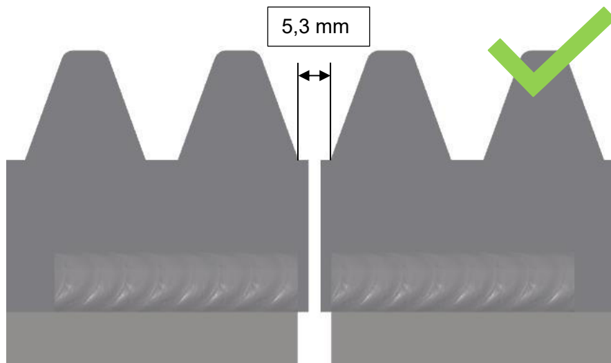
Abbildung 7: Korrekter Abstand.
