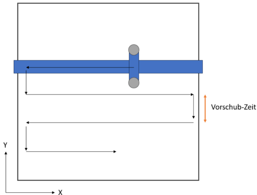
Abbildung 19: Linearfahrt: Modus 2, mit einstellbarer Vorschubzeit
