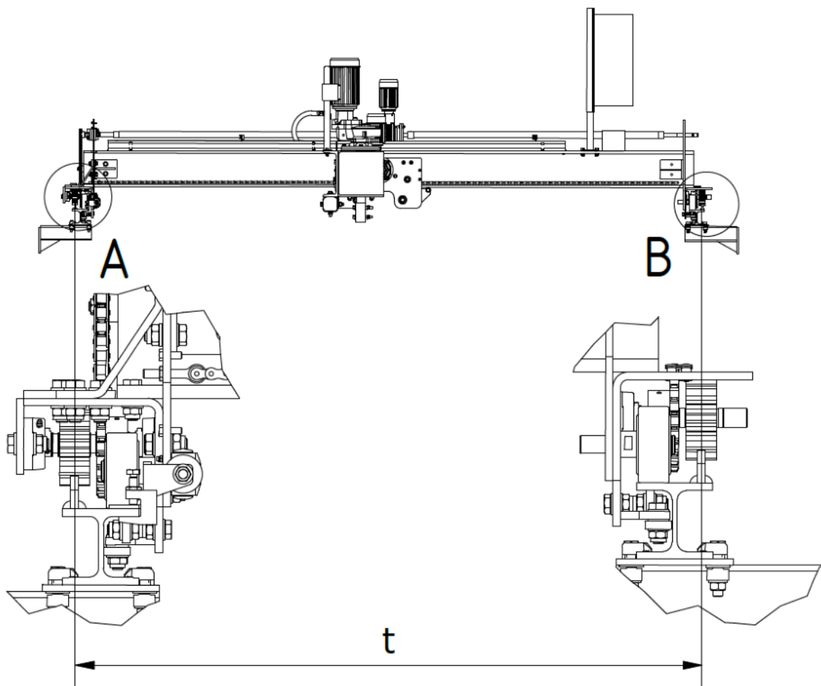
Abbildung 7: Korrekter Abstand.
