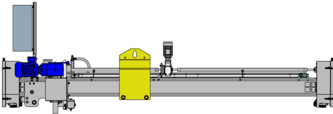
Figura 2: dispositivo de elevación o eslinga de carga opcional (amarilla) para el tornillo mezclador.
