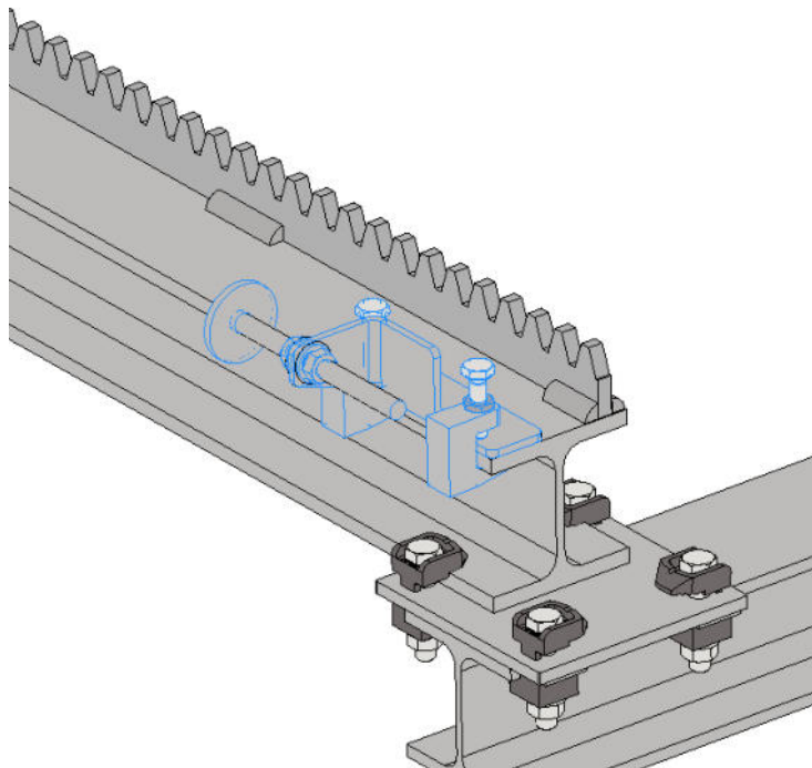
Abbildung 14: Befestigung der Endschalter-Stopper.
