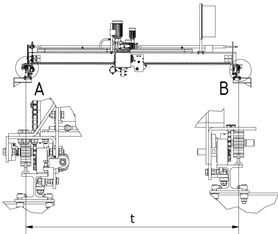
Figura 8: Medición de la distancia t + 10 - 5 mm.
