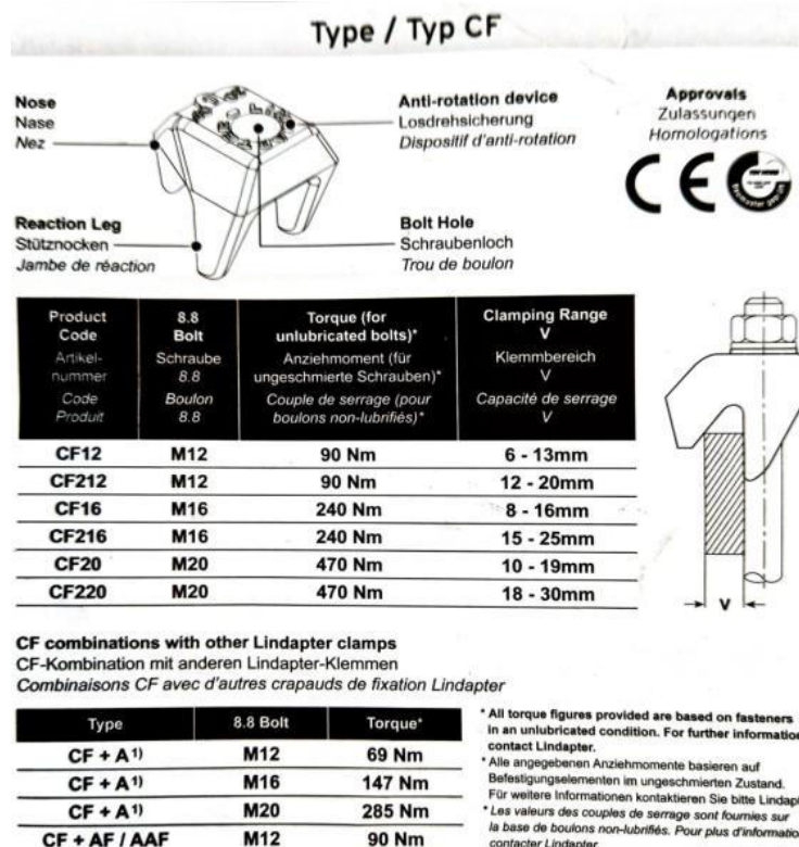
Abbildung 24: Trägerklemmen Typ CF für Laufsteg.
