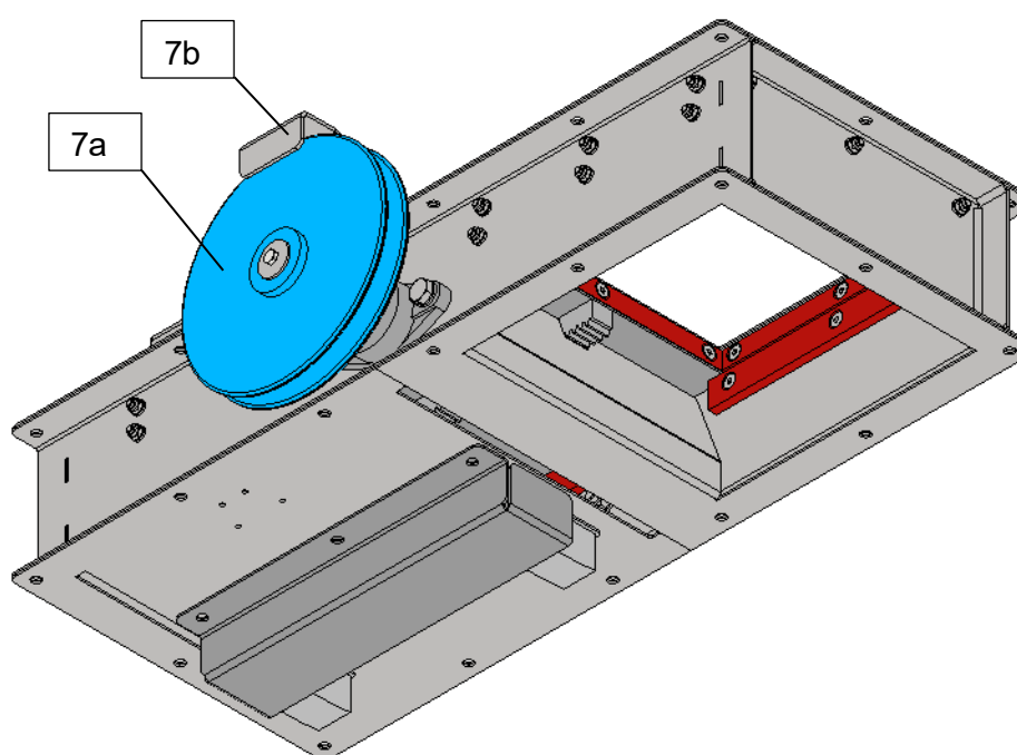
Représentation 3: Vanne avec pignon (vue de dessous)
