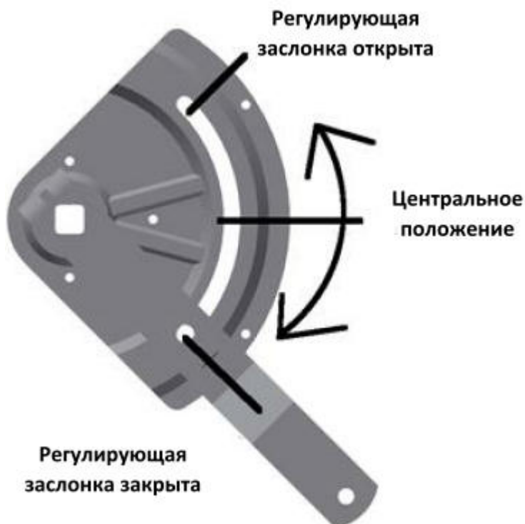
Рис. 6: Положение заслонки (Заслонка - доп. опция)
